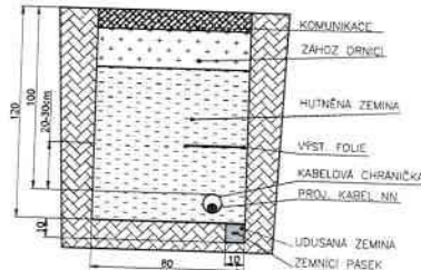
Řez výkopem pod místní a příjezdovou komunikací pro kabel NN a uzemnění (ruční)
