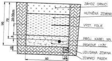
Řez výkopem ve volném terénu pro kabel NN a uzemnění (ruční)
